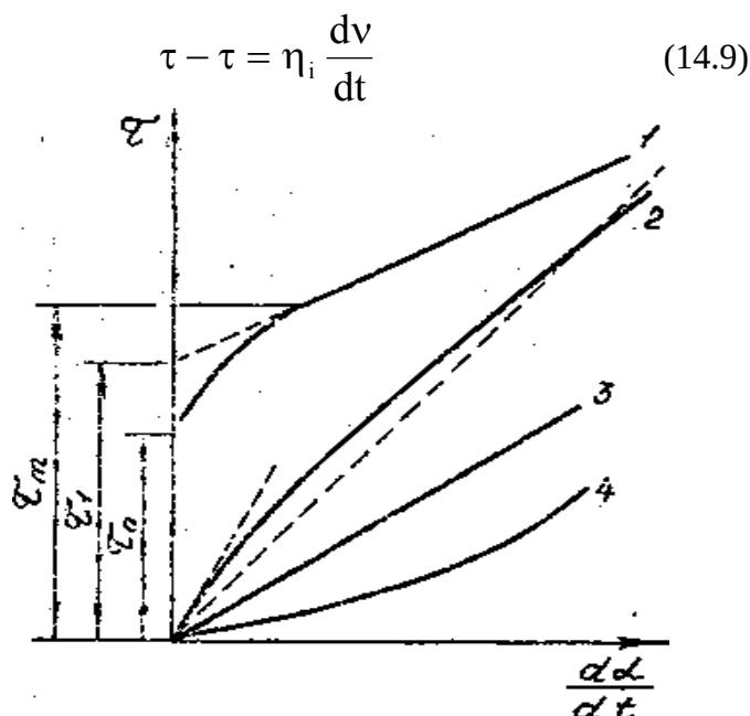
14.3-rasm. Suyuqliklarning konsistentlik bog'liqligi.
