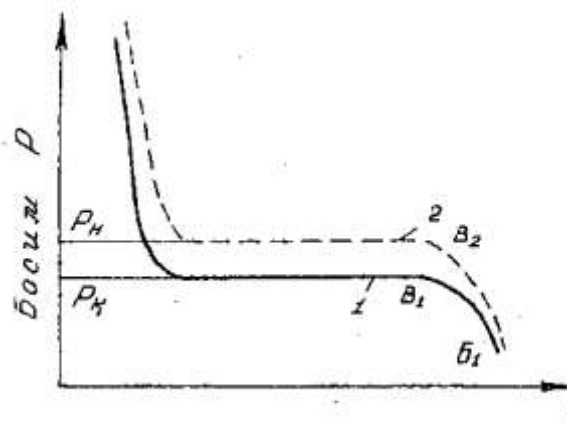
18.2.-rasm. Namlangan uglevodorodlarning fazaviy o'tish grafigi.
