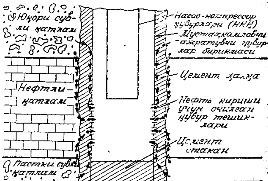
16.1 – rasm. Qudug' tashqarisida qatlam suvlarining xarakat yo'llari.
