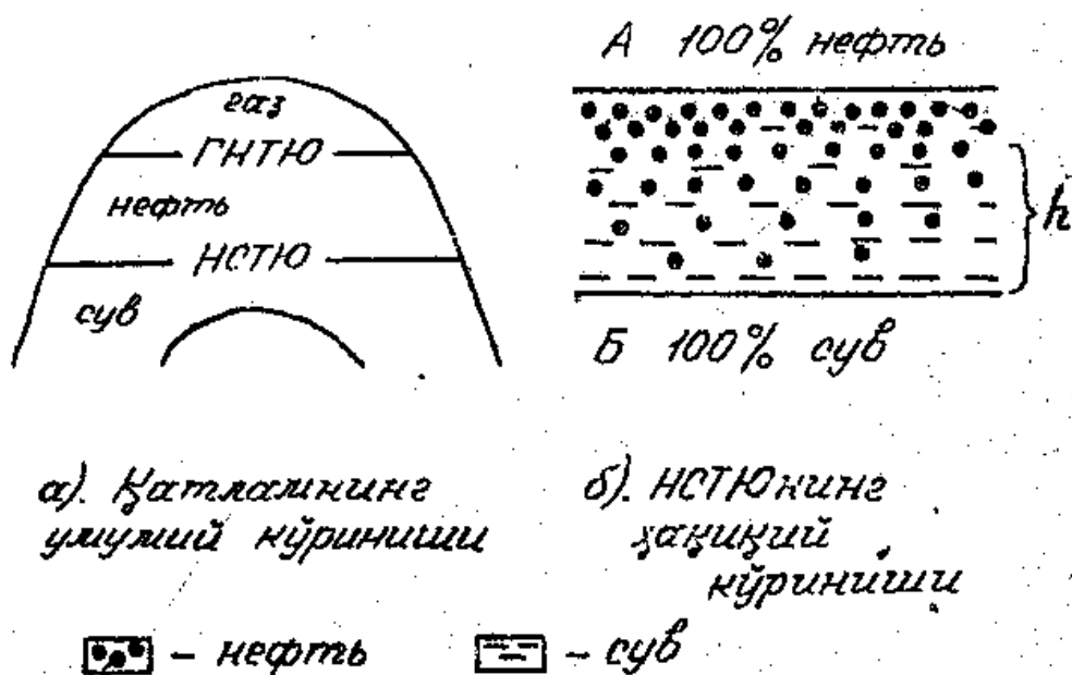
16.2 – rasm. «Neft - suv» tutash yuzasi holati sxemasi
