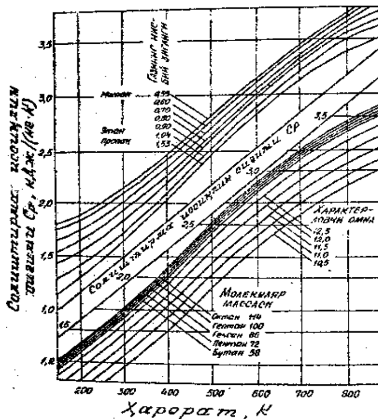
10.7 – rasm. Uglevodorod gazlarining solishtirma issiqlik sig'iminin atmosfera bosimida harorat o'zgarishi bilan bog'liqligi.
