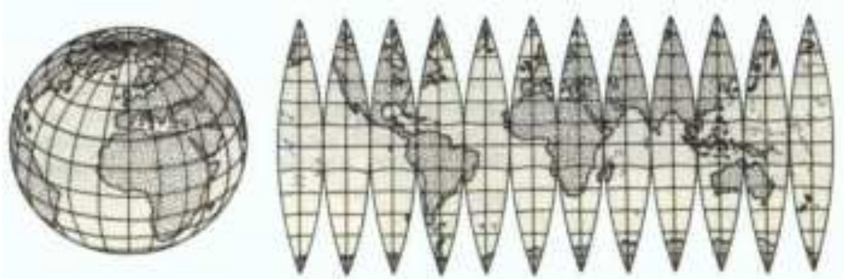
2.3-rasm. Meridianlar bo'yicha zonalarga (tilimlarga) bo'lingan globus yuzasi. Erning egri yuzasini tekislikda uzilishsiz tasvirlab bo'lmavligini tasdiqlovchi sxema
