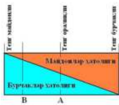
2.7-rasm. Kartografik proeksiyalardagi maydon va burchak xatoliklari o'rtasidagi o'zaro nisbat
